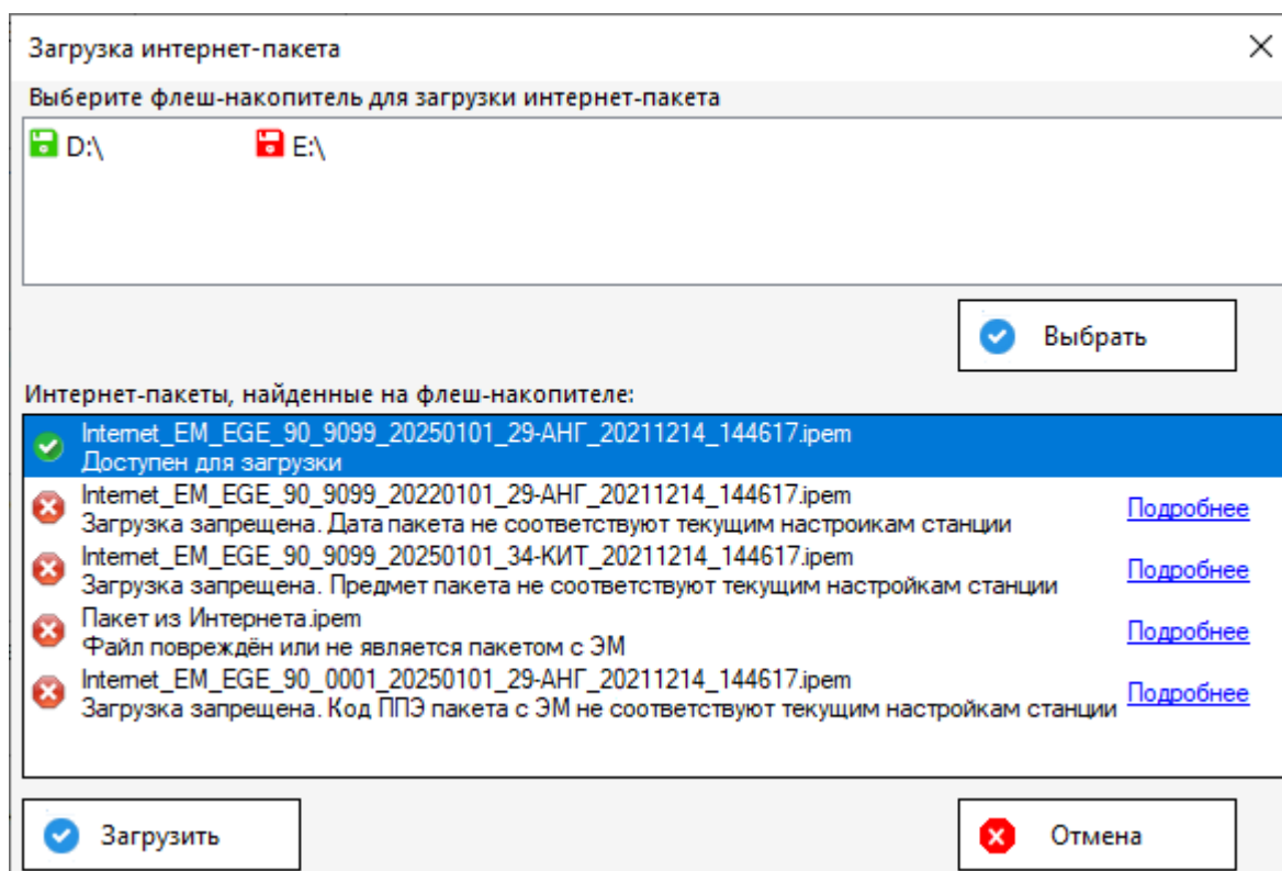
Рис. 6.10. Окно «Загрузка интернет-пакета».
