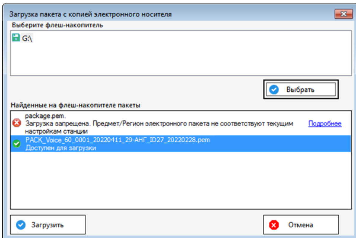
Рис. 8.15. Выбор резервной копии электронного носителя с ЭМ на флеш-накопителе (доставка ЭМ на электронных носителях)
