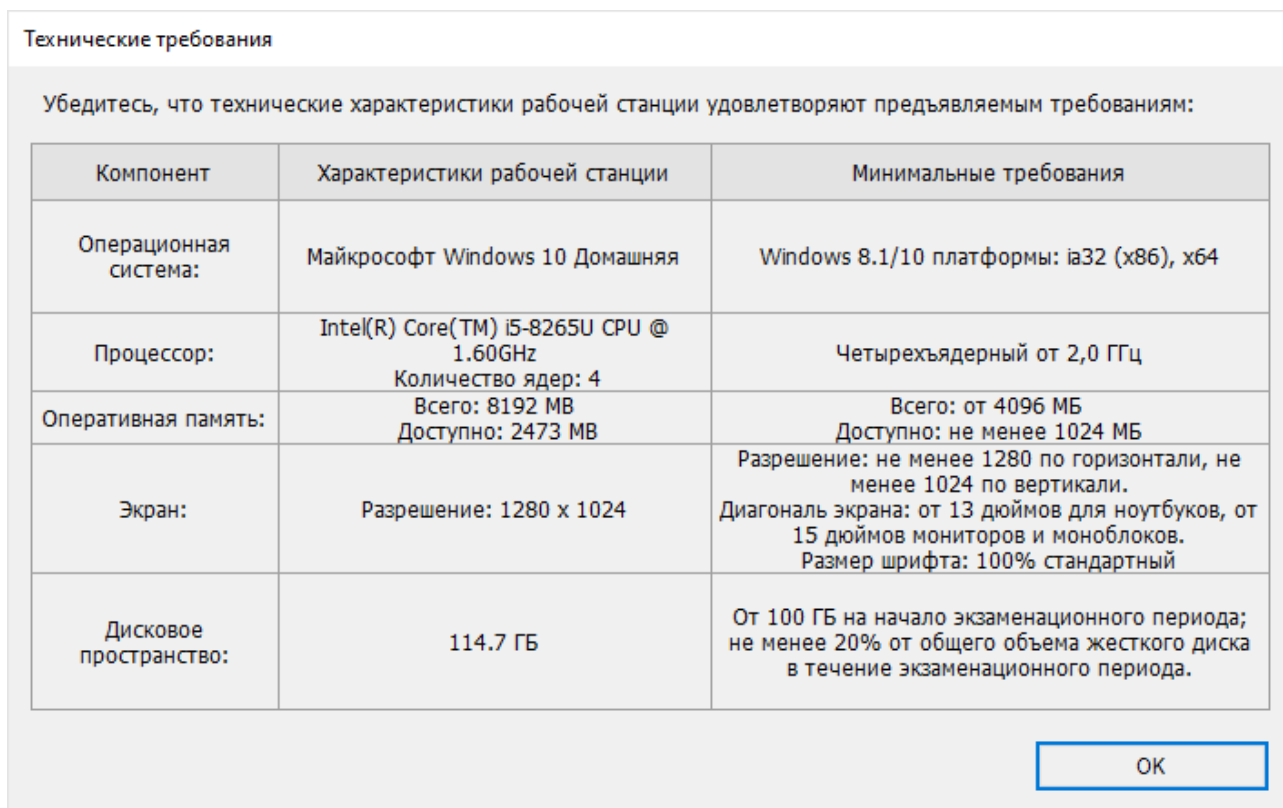
Рис. 6.36. Окно «Технические требования».
