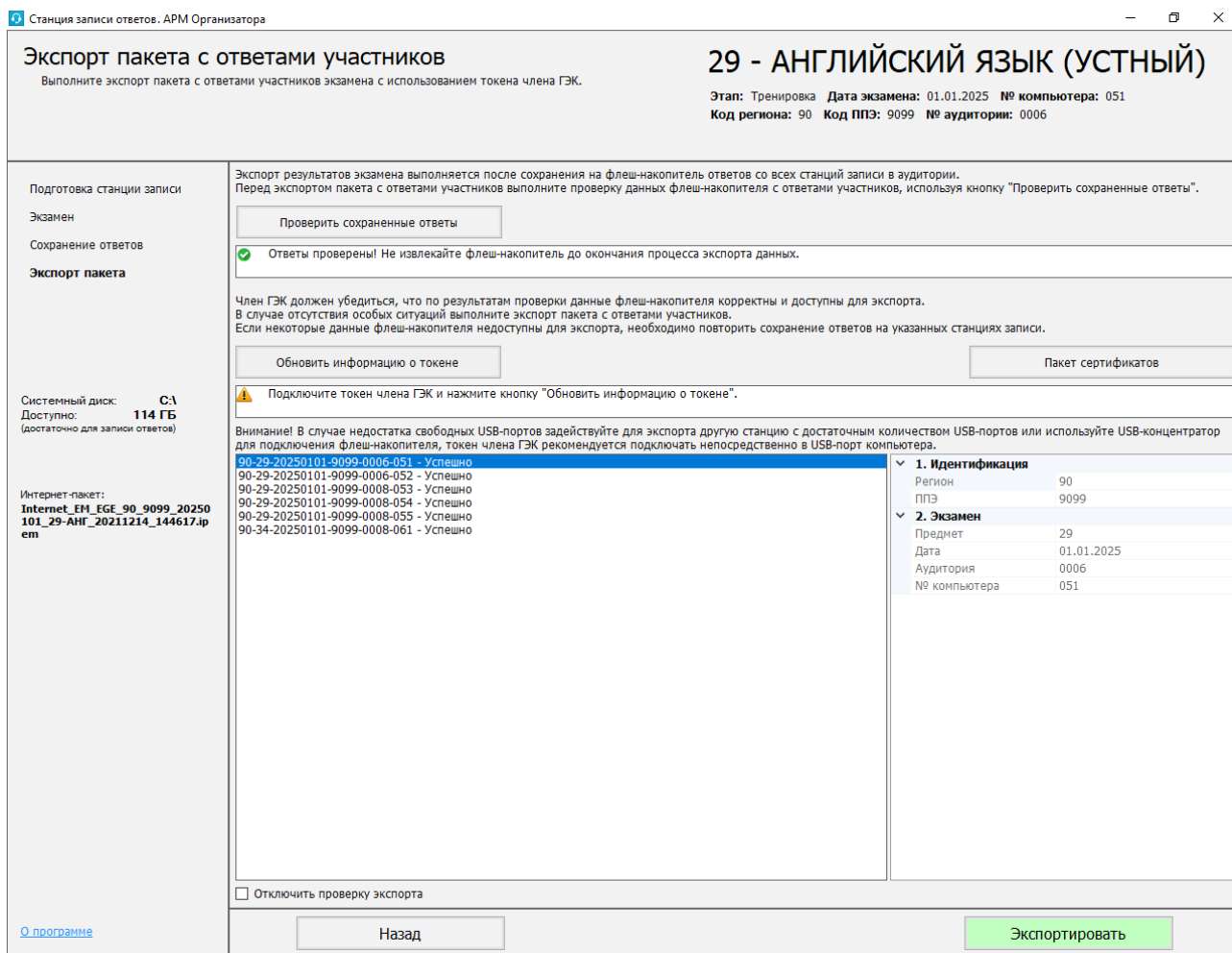
Рис. 11.15. Страница «Экспорт пакета с ответами участников». Флеш-накопитель с ответами проверен успешно.
